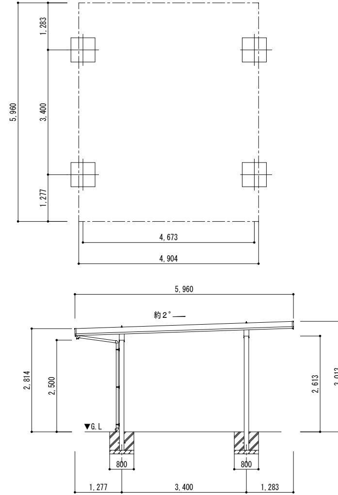
■ 基礎配置図
